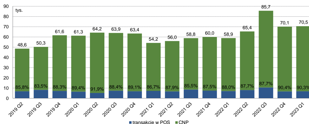
Wykres 15. Struktura liczby bezgotówkowych operacji oszukańczych w okresie od II kwartału 2019 r. do I kwartału 2023 r. w podziale na operacje dokonane w terminalach POS i CNP
