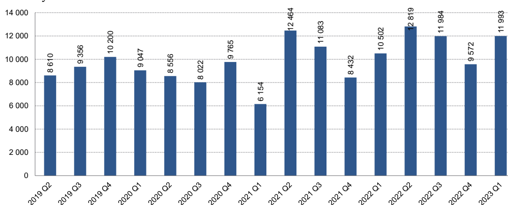
Wykres 4. Liczba operacji oszukańczych przy użyciu kart płatniczych w poszczególnych kwartałach w okresie od II kwartału 2019 r. do I kwartału 2023 r. – dane od agentów rozliczeniowych
