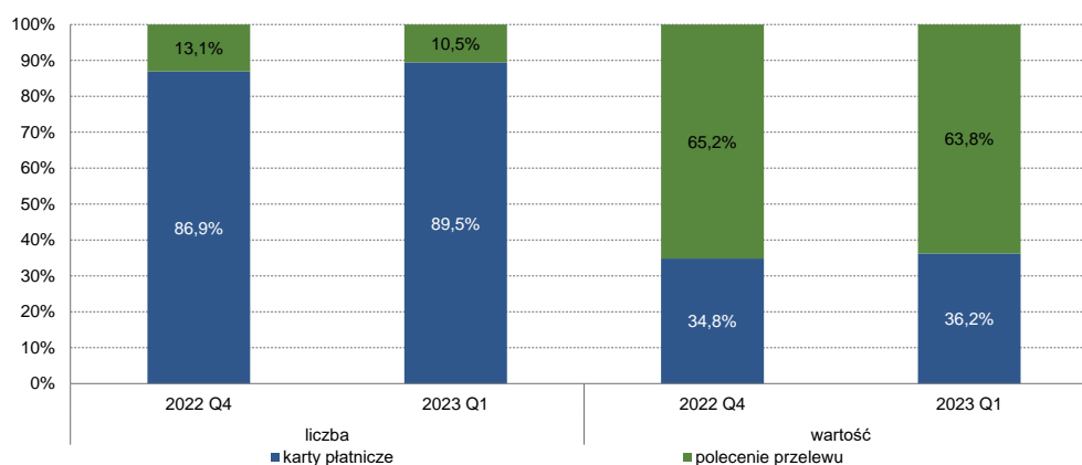
Wykres 2. Struktura operacji oszukańczych przy użyciu poszczególnych bezgotówkowych instrumentów płatniczych według liczby i wartości w IV kwartale 2022 r. oraz I kwartale 2023 r. – dane od banków
