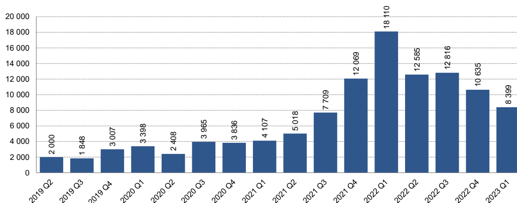
Wykres 19. Liczba operacji oszukańczych z wykorzystaniem polecenia przelewu w okresie od II kwartału 2019 r. do I kwartału 2023 r. w podziale na poszczególne kwartały
