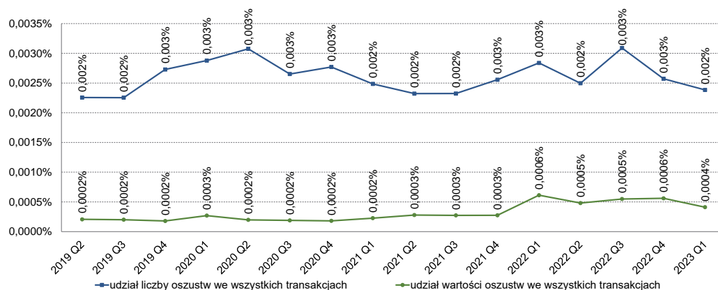
Wykres 1. Udział procentowy liczby i wartości oszustw we wszystkich transakcjach kartami płatniczymi oraz poleceniach przelewu w okresie od II kwartału 2019 r. do I kwartału 2023 r. – dane od banków
