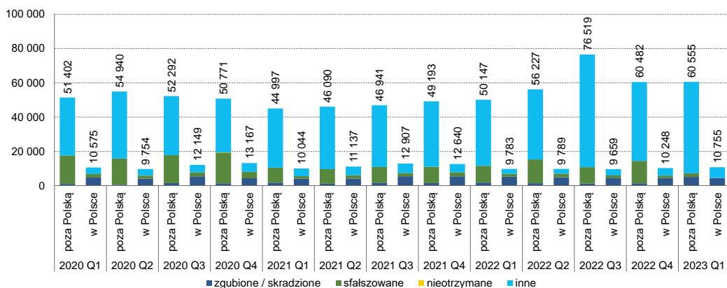
Wykres 13. Struktura operacji oszukańczych kartami płatniczymi w podziale na rodzaje oszustw według liczby transakcji w okresie od I kwartału 2020 r. do I kwartału 2023 r. – dane od banków
