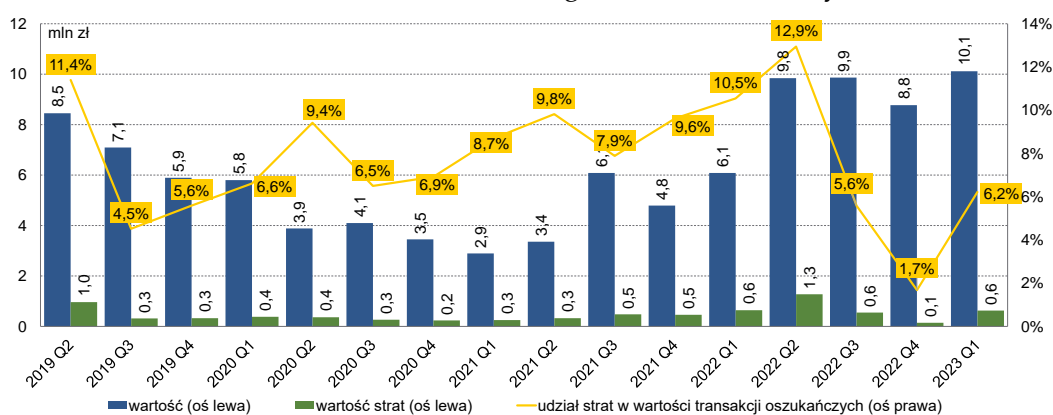
Wykres 5. Wartość operacji oszukańczych przy użyciu kart płatniczych oraz wartość strat poniesionych przez agentów rozliczeniowych w poszczególnych kwartałach w okresie od II kwartału 2019 r. do I kwartału 2023 r. – dane od agentów rozliczeniowych
