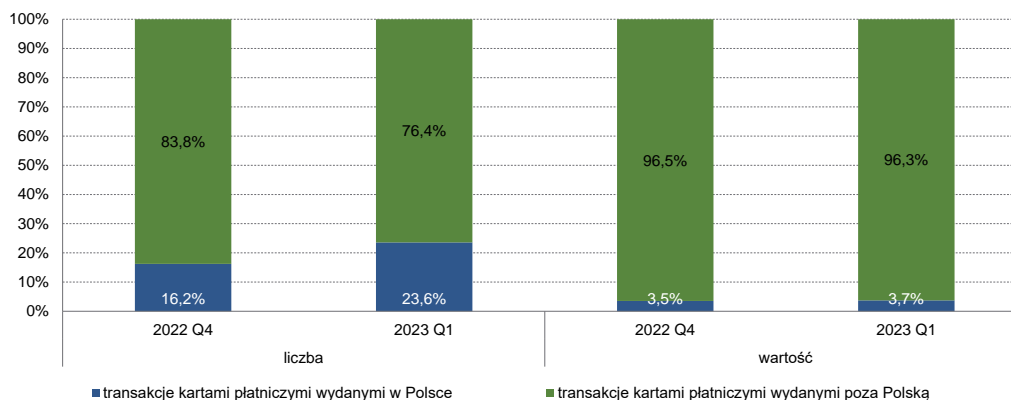
Wykres 7. Struktura operacji oszukańczych przy użyciu kart płatniczych według liczby i wartości w IV kwartale 2022 r. oraz I kwartale 2023 r. – dane od agentów rozliczeniowych
