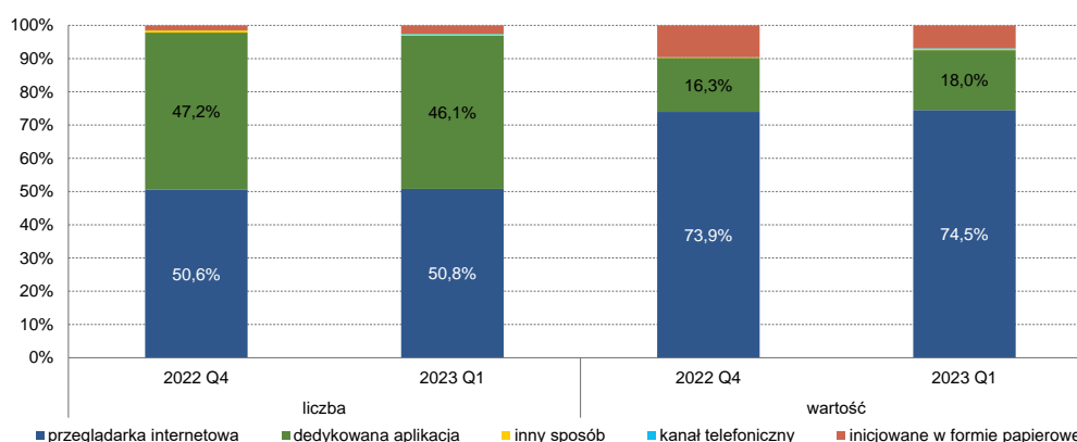
Wykres 21. Struktura operacji oszukańczych przy użyciu polecenia przelewu według liczby i wartości w IV kwartale 2022 r. oraz I kwartale 2023 r. – dane od banków
