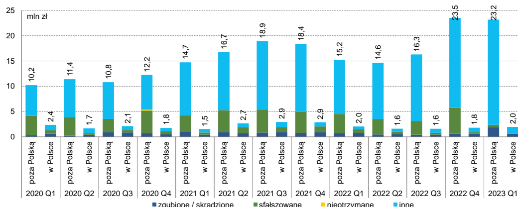
Wykres 14. Struktura operacji oszukańczych kartami płatniczymi w podziale na rodzaje oszustw według wartości transakcji w okresie od I kwartału 2020 r. do I kwartału 2023 r. – dane od banków
