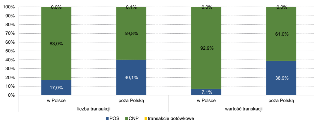
Wykres 8. Struktura transakcji oszukańczych przy użyciu kart płatniczych w POS, CNP i gotówkowych ogółem – liczba i wartość transakcji – I kwartał 2023 r.
