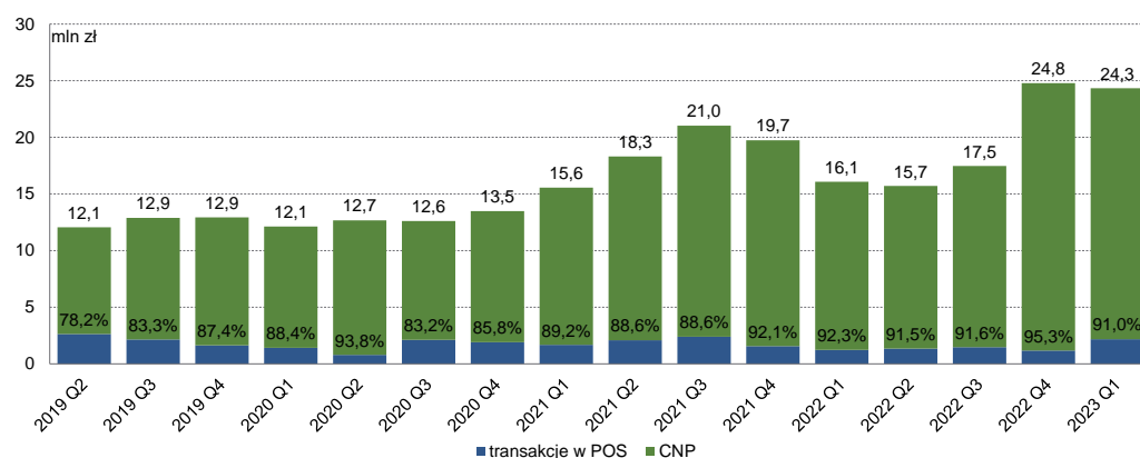
Wykres 16. Struktura wartości bezgotówkowych operacji oszukańczych w okresie od II kwartału 2019 r. do I kwartału 2023 r. w podziale na operacje dokonane w terminalach POS i CNP
