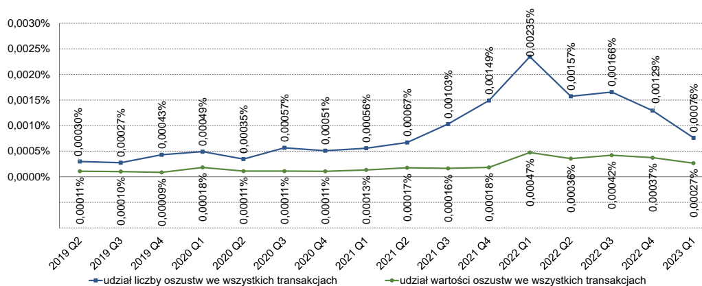
Wykres 20. Udział procentowy liczby i wartości oszustw we wszystkich transakcjach polecenia przelewu w okresie od II kwartału 2019 r. do I kwartału 2023 r. – dane od banków
