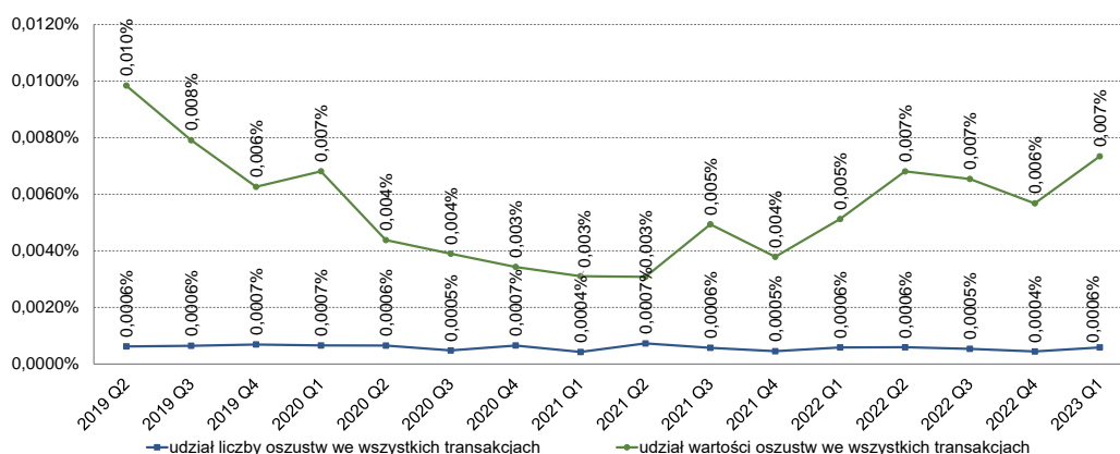
Wykres 6. Udział procentowy liczby i wartości oszustw we wszystkich transakcjach kartami płatniczymi w okresie od II kwartału 2019 r. do I kwartału 2023 r. – dane od agentów rozliczeniowych
