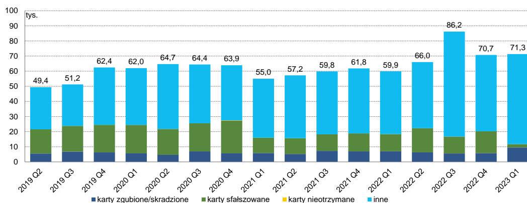
Wykres 11. Liczba operacji oszukańczych przy użyciu kart płatniczych w poszczególnych kwartałach w okresie od II kwartału 2019 r. do I kwartału 2023 r. w podziale na rodzaje operacji oszukańczych – dane od banków
