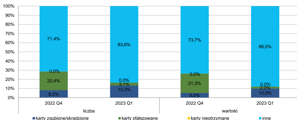
Wykres 10. Struktura operacji oszukańczych kartami płatniczymi według liczby i wartości w IV kwartale 2022 r. oraz I kwartale 2023 r. – dane od banków
