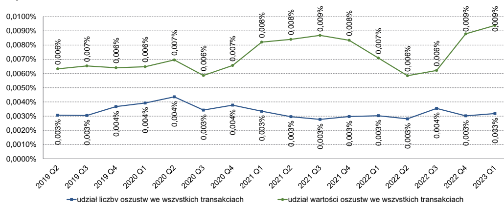
Wykres 17. Udział procentowy liczby i wartości oszustw we wszystkich transakcjach kartami płatniczymi w okresie od II kwartału 2019 r. do I kwartału 2023 r. – dane od banków
